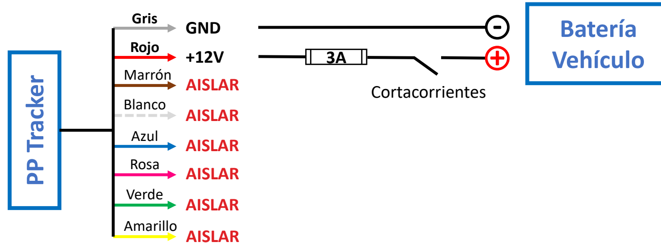
Imagen 7. ESQUEMA DE CONEXIÓN ELÉCTRICA PPTRACKER
