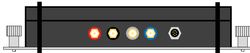
Imagen 8. ESQUEMA DE CONEXIONES TERMINALES PPTRACKER
